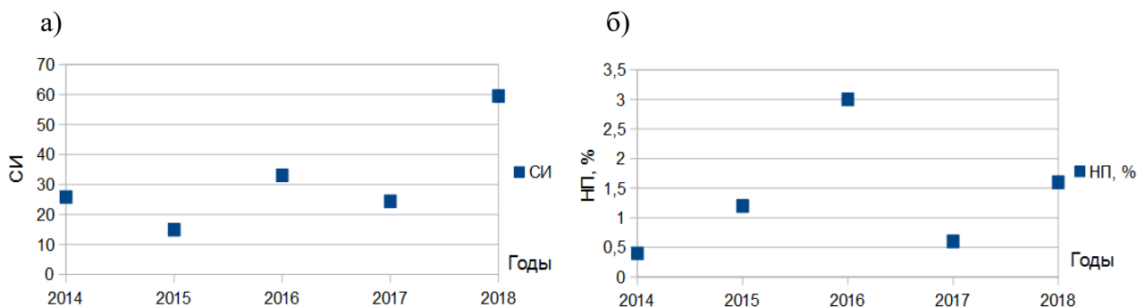
Рисунок 1.23 Изменение показателей загрязнения атмосферы в г. Лесосибирск за период 2014-2018 гг.: а) – СИ, б) – НП.
