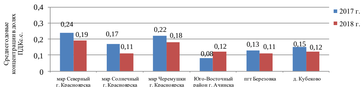
Рисунок 1.8 Среднегодовые концентрации оксида углерода в долях ПДКс.с. в 2017 и 2018 гг.
