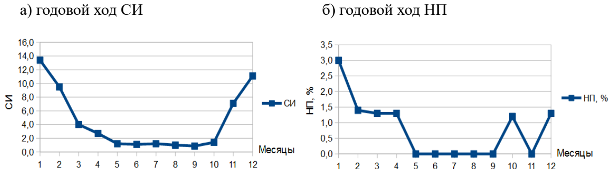
Рисунок 1.18 Годовой ход показателей загрязнения атмосферы в г. Ачинск
