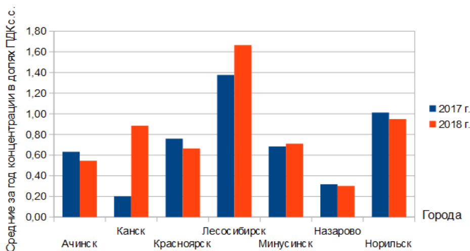
Рисунок 1.1 Среднегодовые концентрации взвешенных веществ в долях ПДК с.с. в 2017 и 2018 гг.
