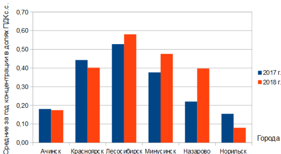
Рисунок 1.2 Среднегодовые концентрации оксида углерода в долях ПДК с.с. в 2017 и 2018 гг.
