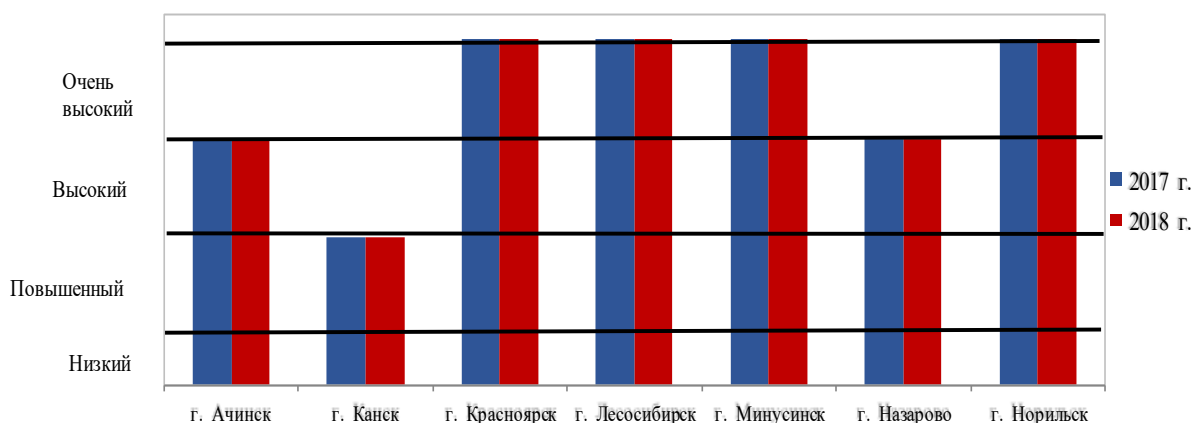
Рисунок 1.15 Уровень загрязнения атмосферного воздуха городов Красноярского края в 2017 и 2018 гг. по результатам наблюдений ФГБУ «Среднесибирское УГМС»
