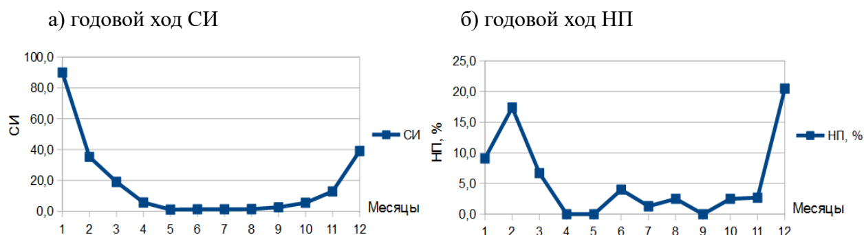
Рисунок 1.24 Годовой ход показателей загрязнения атмосферы в г. Минусинск
