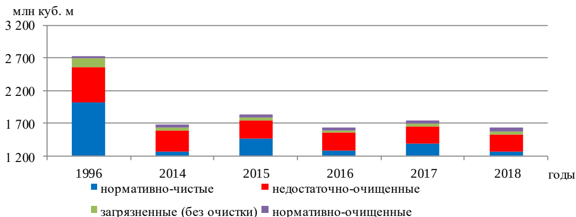
Рисунок 4.3 Объемы и категории сточных вод, сбрасываемых в поверхностные водные объекты (1996, 2014-2018 гг.)
