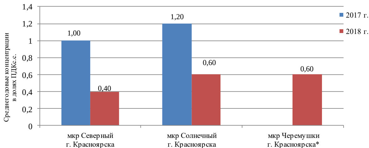
Рисунок 1.12 Среднегодовые концентрации гидрофторида в долях ПДК с.с. в 2017 и 2018 гг.
