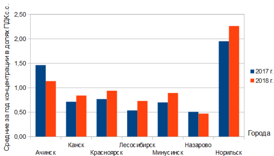
Рисунок 1.3 Среднегодовые концентрации диоксида азота в долях ПДК с.с. в 2017 и 2018 гг.
