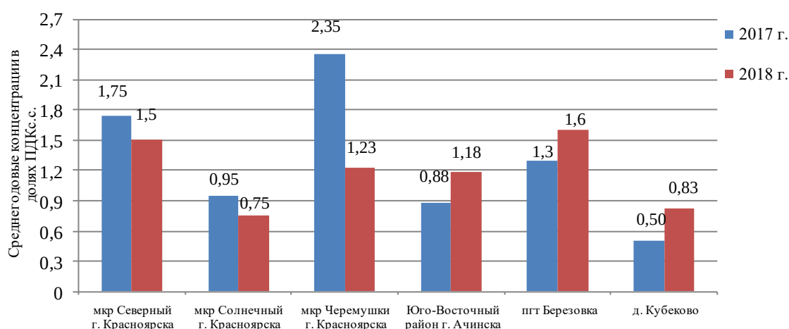
Рисунок 1.9 Среднегодовые концентрации диоксида азота в долях ПДКс.с. в 2017 и 2018 гг.
