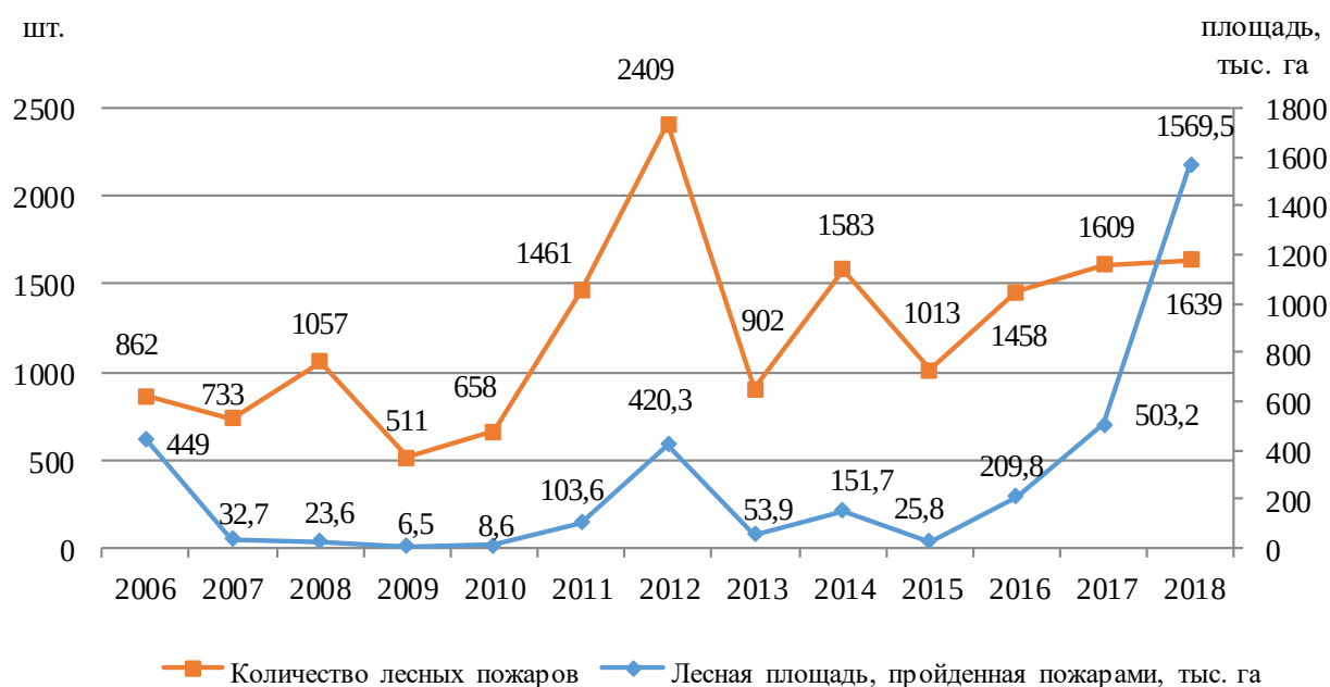
Рисунок 1.13 Динамика лесных пожаров и площадь, пройденная пожарами в крае за 2006-2018 гг.
