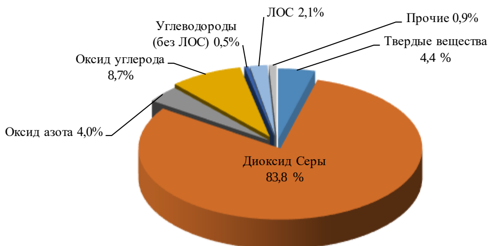
Рисунок 1.30 Состав выбросов загрязняющих веществ от стационарных источников
