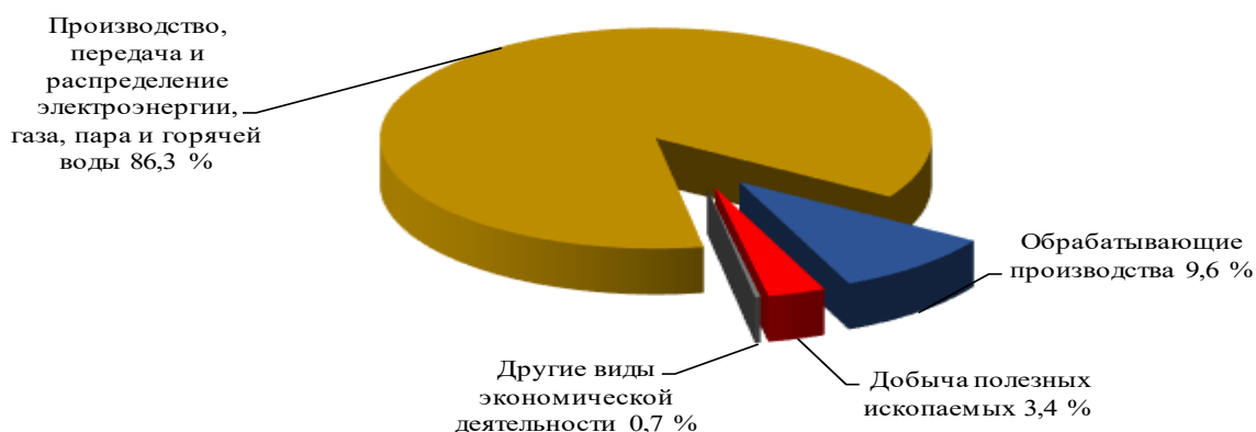
Рисунок 12.2 Доля видов экономической деятельности в объеме сбросов сточных вод в поверхностные водные объекты в 2018 г.
