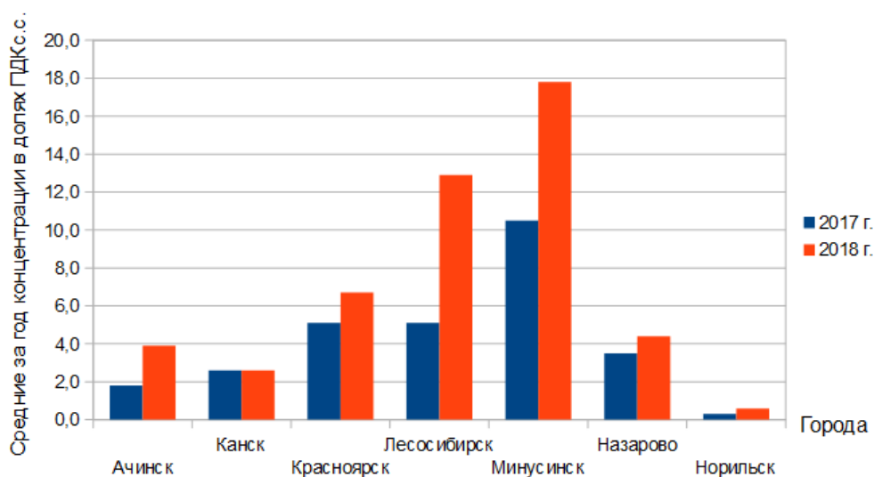
Рисунок 1.5 Среднегодовые концентрации бенз(а)пирена в долях ПДК с.с. в 2017 и 2018 гг.
