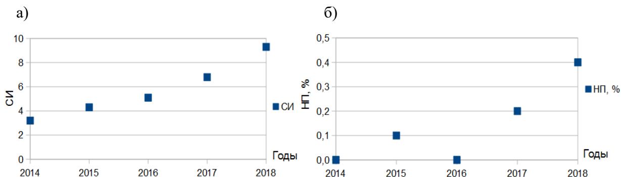
Рисунок 1.21 Изменение показателей загрязнения атмосферы в г. Канск за период 2014-2018 гг.: а) – СИ, б) – НП.
