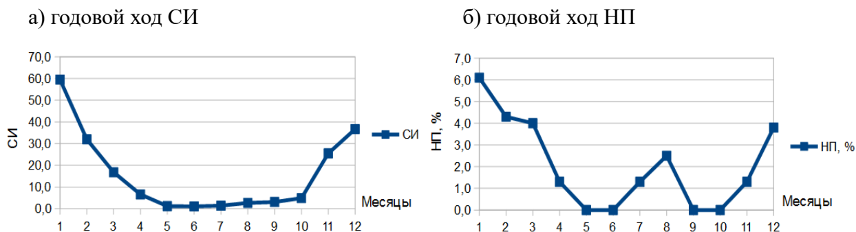
Рисунок 1.22 Годовой ход показателей загрязнения атмосферы в г. Лесосибирск
