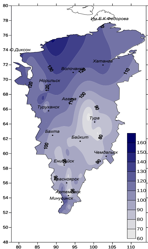
Рисунок. 3.2. Аномалии годового количества осадков, %
