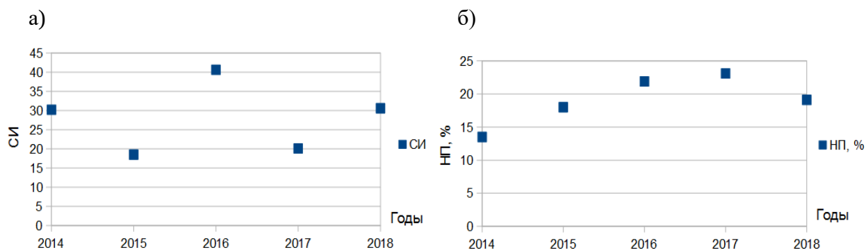
Рисунок 1.17 Изменение показателей загрязнения атмосферы в г. Красноярск за период 2014-2018 гг.: а) – СИ, б) – НП.
