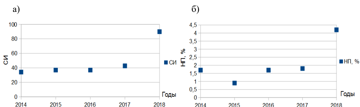
Рисунок 1.25 Изменение показателей загрязнения атмосферы в г. Минусинск за период 2014-2018 гг.: а) – СИ, б) – НП.
