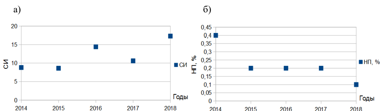
Рисунок 1.27 Изменение показателей загрязнения атмосферы в г. Назарово за период 2014-2018 гг.: а) – СИ, б) – НП.
