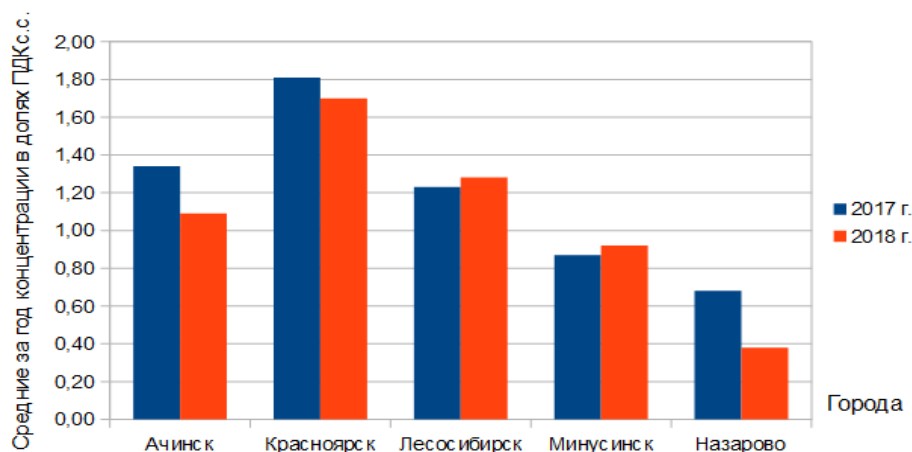
Рисунок 1.6 Среднегодовые концентрации формальдегида в долях ПДК с.с. в 2017 и 2018 гг.
