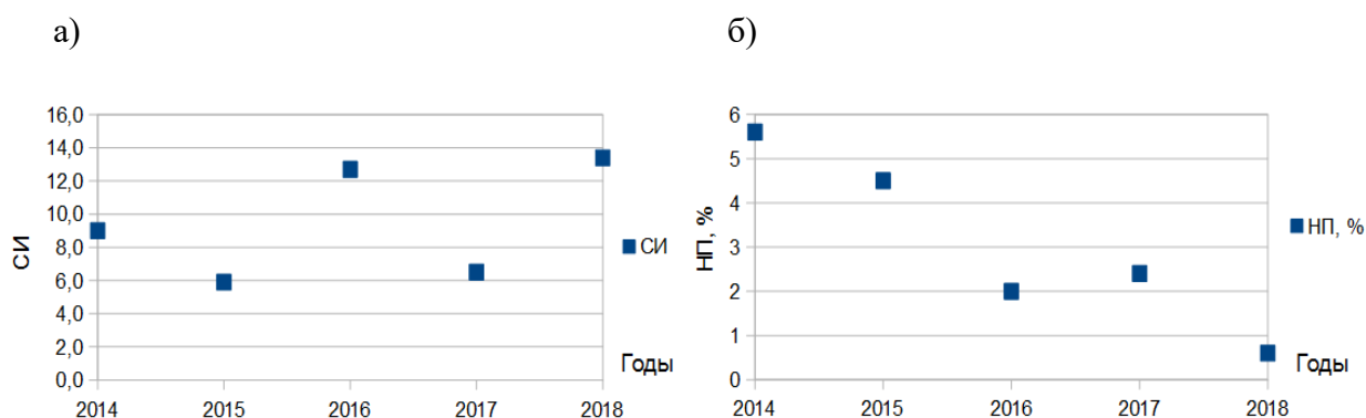
Рисунок 1.19 Изменение показателей загрязнения атмосферы в г. Ачинск за период 2014-2018 гг.: а) – СИ, б) – НП.
