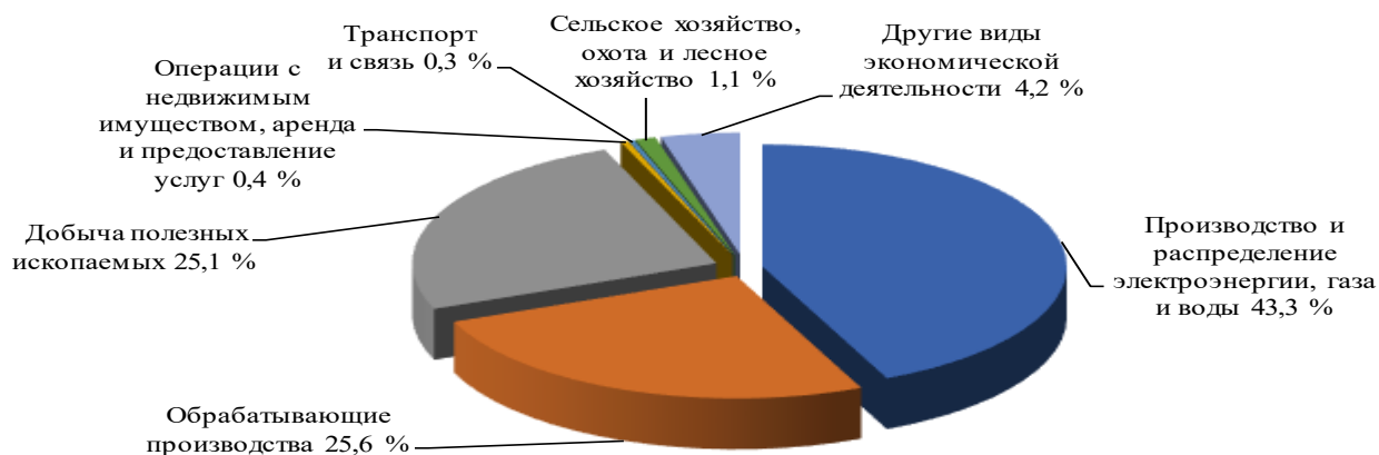
Рисунок 12.1 Выбросы загрязняющих веществ в атмосферу от стационарных источников отраслей промышленности края (без учета выбросов ЗФ ПАО «ГМК «Норильский никель») в 2018 г.
